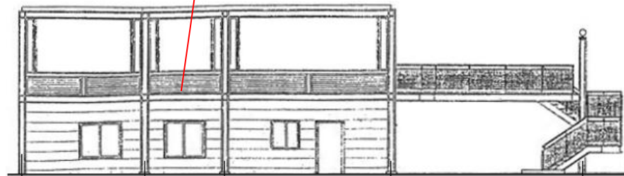
南立面図
